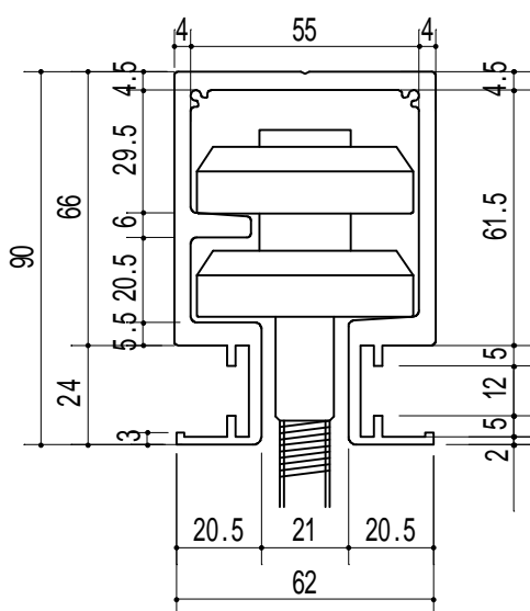
型材断面詳細図 (1/2)
