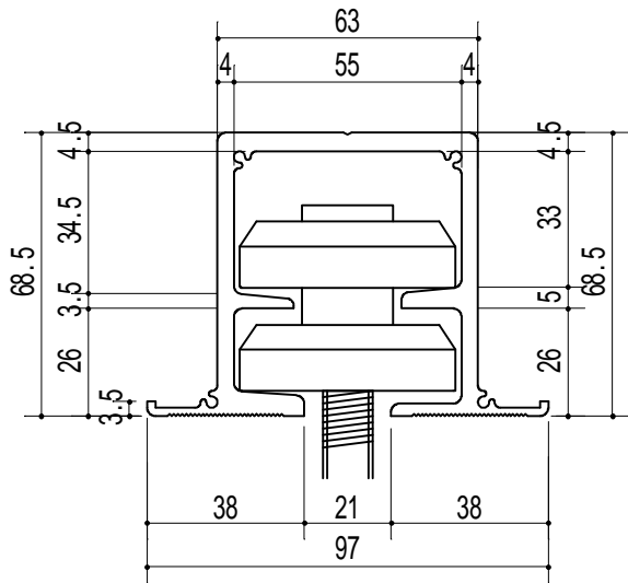
型材断面詳細図(1/2)
