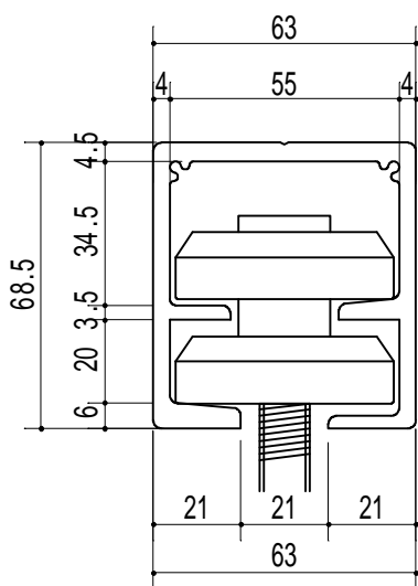
型材断面詳細図(1/2)
