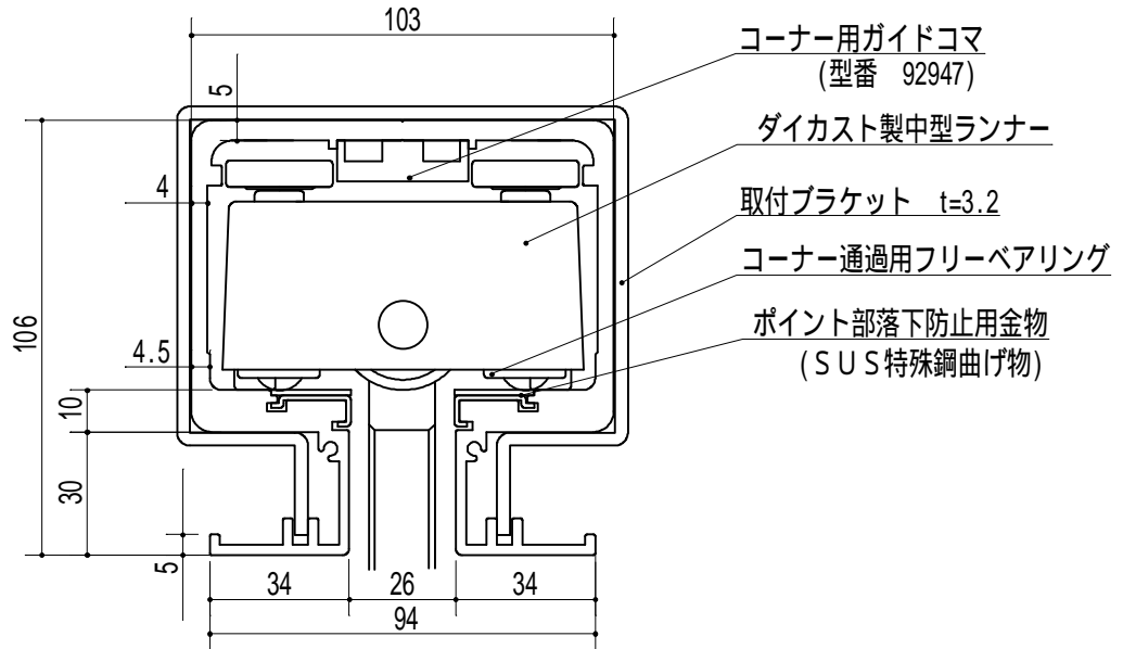
型材断面詳細図 (1/2) (ランナー: FB式)
