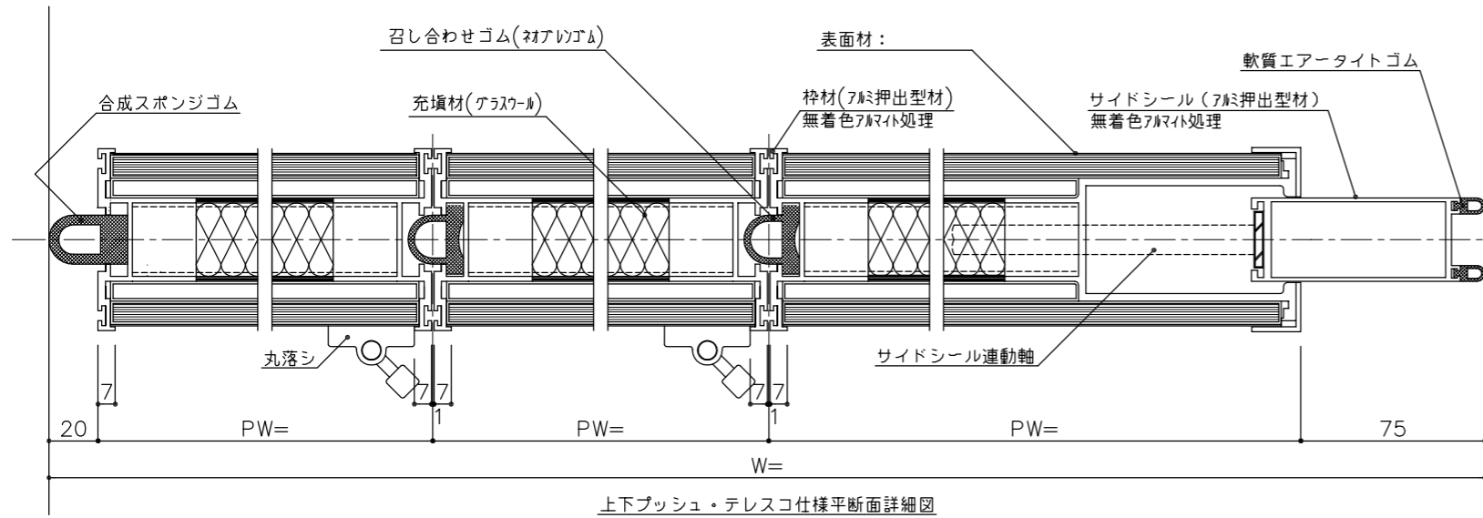
上下プッシュ・テレスコ仕様断面詳細図
