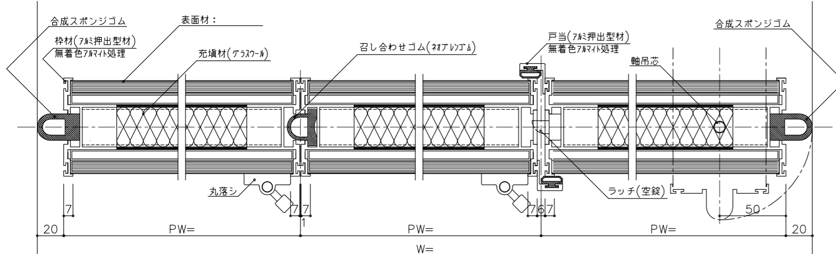
蝶番仕様断面詳細図
