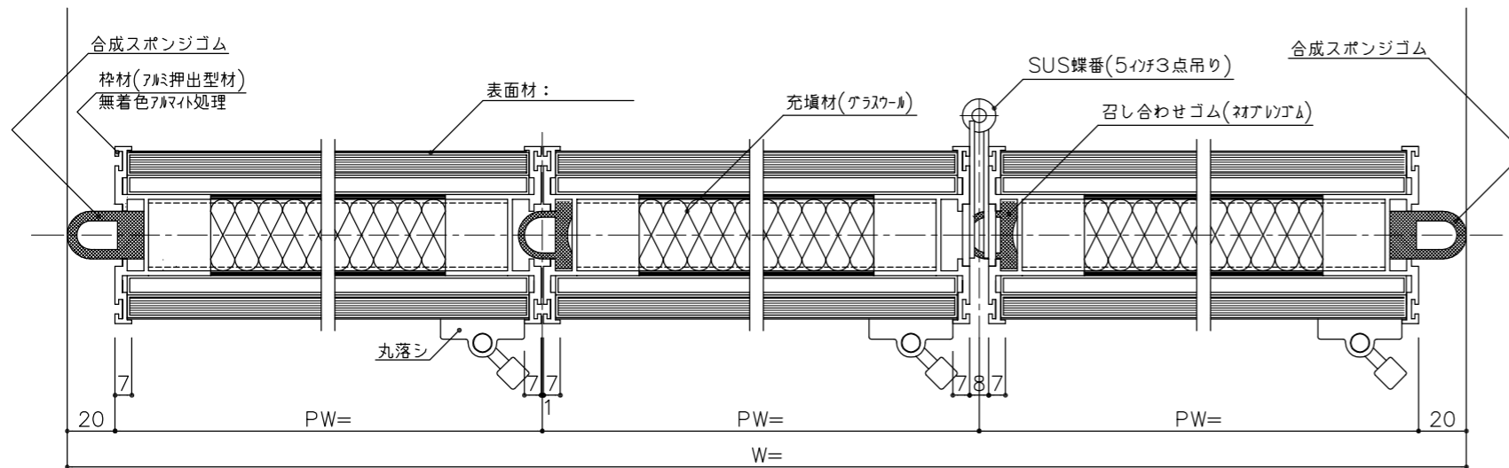
蝶番仕様断面詳細図
